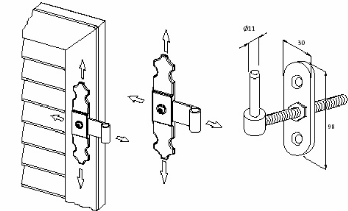
HINGES
